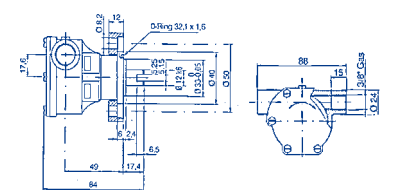
16.00135 ST135 Bocche da 3/8, portata lt./min. 13/28 per motori Ruggerini, Lombardini, Nanni, Mitsubishi, Lister Petter, Watermota.
