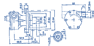
16.00136 ST136 Bocche da 3/8, portata lt./min. 13/28 per motori Vetus K.
