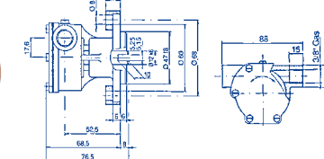
16.00138 ST138 Bocche da 3/8, portata lt./min. 13/28 per motori Lombardini LDW 903, Aifo 4041, Volvo Penta AQ-BB-MB-MDI-2000
