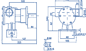
16.00040 PM 40 Bocche da 1' 1/2, portata lt./min. 95/293
