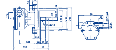
16.00139 ST139 Bocche da 3/8, portata lt./min. 13/28 per motori Lombardini, Aifo.
