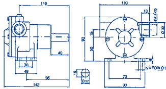
16.00034 PM 34 Bocche da 3/4, portata lt./min. 18/49
