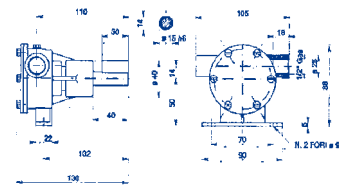
16.00016 PM 16 Bocche da 1/2, portata lt./min. 17,5/50
