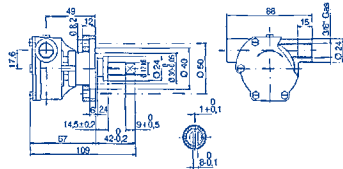
16.00134 ST134 Bocche da 3/8, portata lt./min. 13/28 per motori Vetus M.
