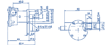
16.00114 ST114 Bocche da 3/8, portata lt./min. 7/14 per motori Volvo Penta, Bukh, Arona, Ducati, Ruggerini, Nanni ecc...
