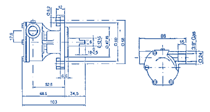
16.00137 ST137 Bocche da 3/8, portata lt./min. 13/28 per motori Nanni FK2/ FK3, Aifo, Mitsubishi.
